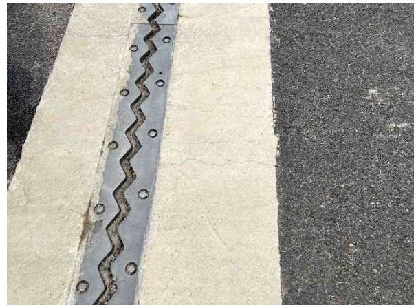
신축이음 A2 후타재 균열(Cw=0.3mm미만)
