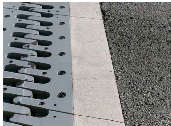
A1 후타재 균열( C_w=0.3\text{mm} 미만)
