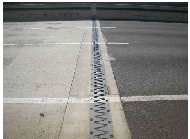
A1 접속부 이격(13.0m)
