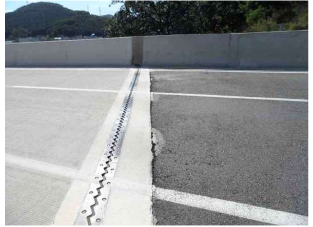
신축이음 전경(문산)
