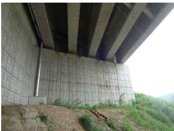
교대 전경(서울)
