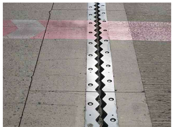
A1 후타재 (0.2mm/0.4m×17EA)
