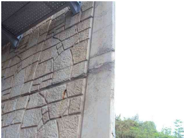
교대 A1 재료분리(0.3×0.3×2EA)
