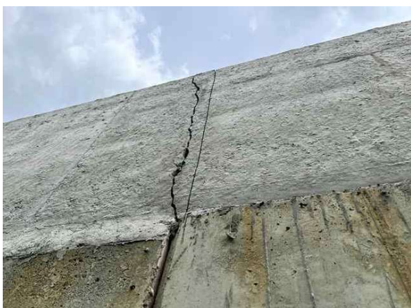
방호벽 S1 접속부 파손(0.1 × 1.5)
