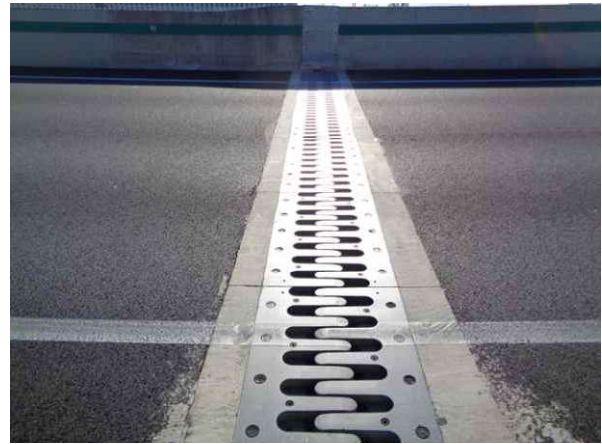
P0 상태양호
