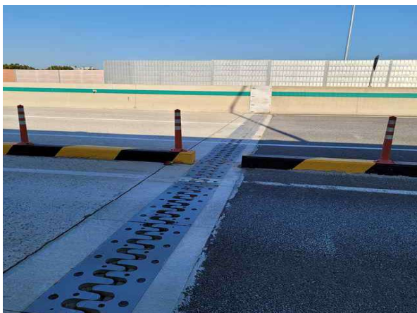
S7 접속부 이격(12.0m)
