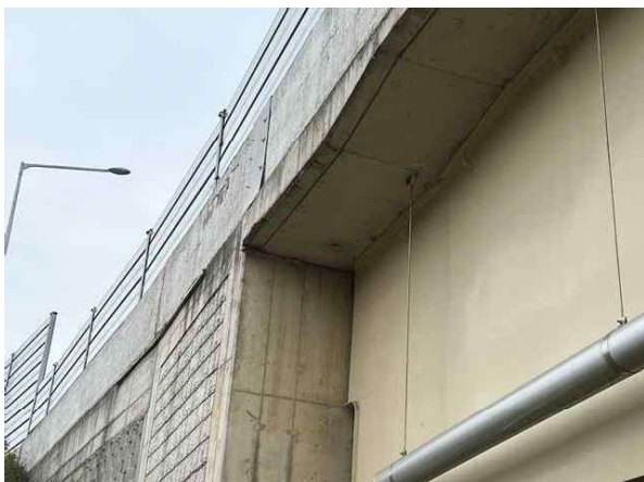
바닥판 하면 S1 백태(0.3×0.3)
