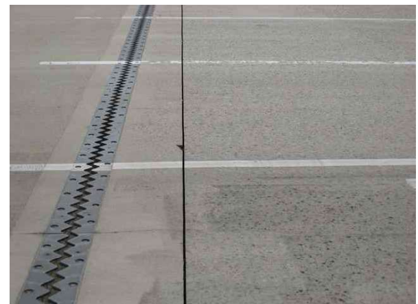
A1 후타재 파손 - 22년 상반기
