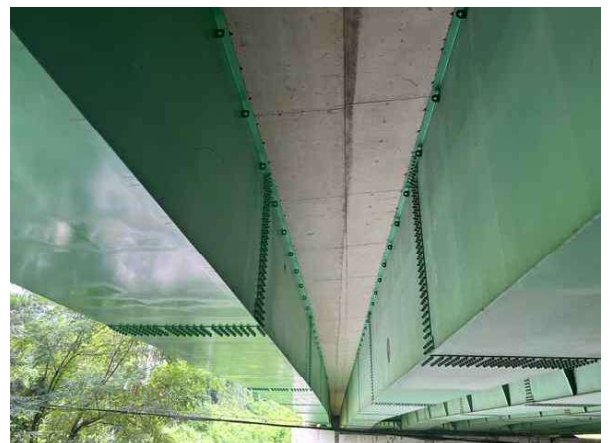
바닥판하면 전경
