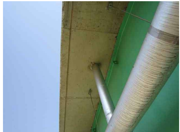
바닥판 하면 S4 상태양호
